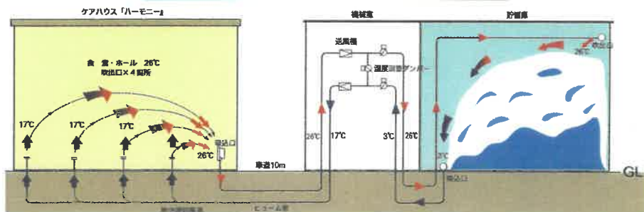
ケアハウス「ハーモニー」雪冷房システム図
